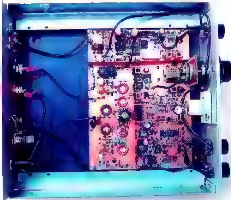
Binnenwerk 40 meterzendontvanger. Alles op een mooi printontwerp (Duits ontwerp).
